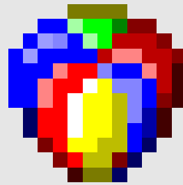
= OpaqueImage
